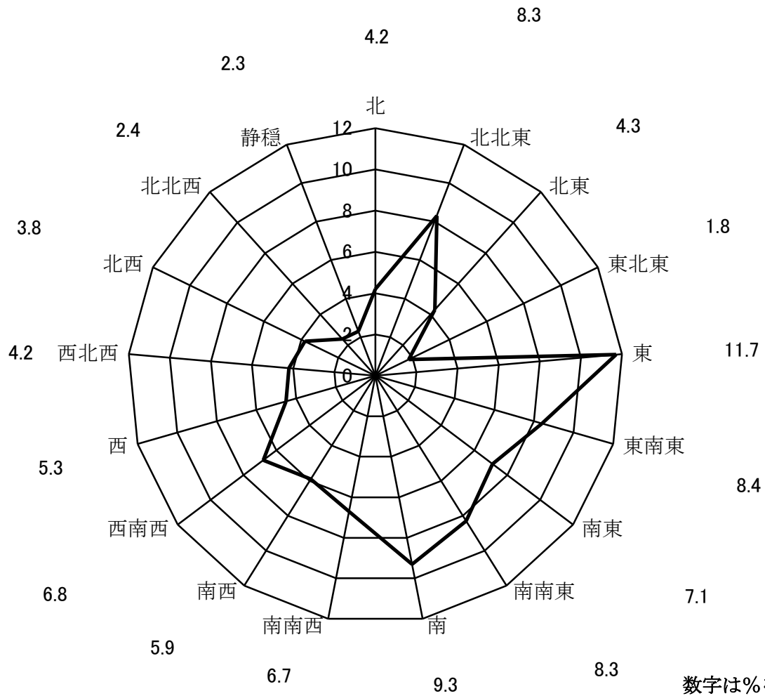
風向頻度
