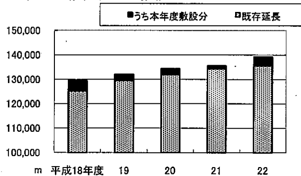
消雪パイプ敷設状況の推移
