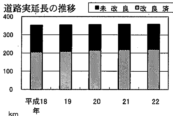
舗装状況の推移
